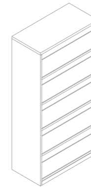
Model : JT-ZZ-2100 Name : 单面杂志架 Size : 900W × 450D × 2100H
