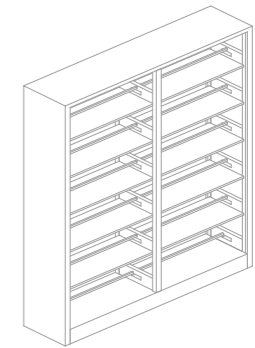
Model : JT-TS-2000 Name : 双面书架 Size : 1900W × 450D × 2000H
